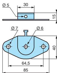
Flange: 79696042
